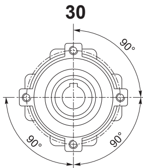
4 Fori / HoleОтверстия
