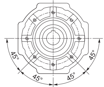
8 Fori / HoleОтверстия
